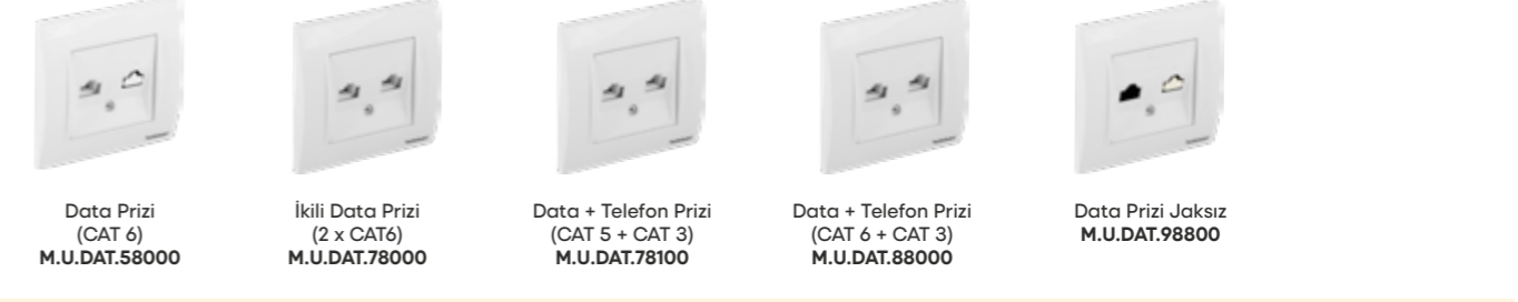
Numeris Telefon Prizi (RJ11) M.U.DAT.18600 İkili Numeris Telefon Prizi (2 x RJ11) M.U.DAT.18700 Numeris Telefon Prizi (CAT 3) M.U.DAT.18000 İkili Numeris Telefon Prizi (2 x CAT 3) M.U.DAT.28000 Data Prizi (CAT5) M.U.DAT.38000 İkili Data Prizi (2 x CAT5) M.U.DAT.48000
