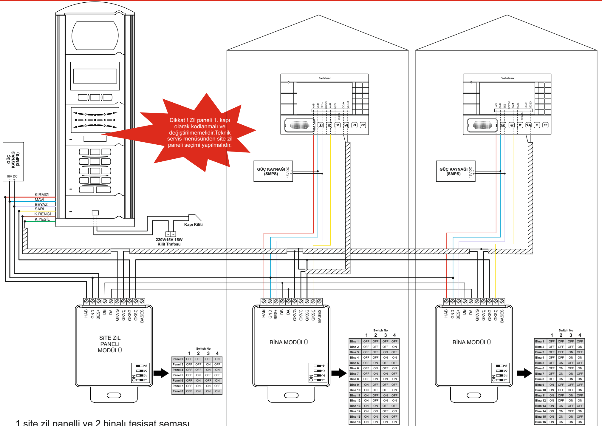
1 site zil paneli ve 2 binalı tesisat şeması
